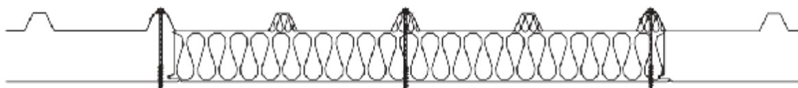
Рис. 2 Размещение самонарезающих винтов с наездниками
