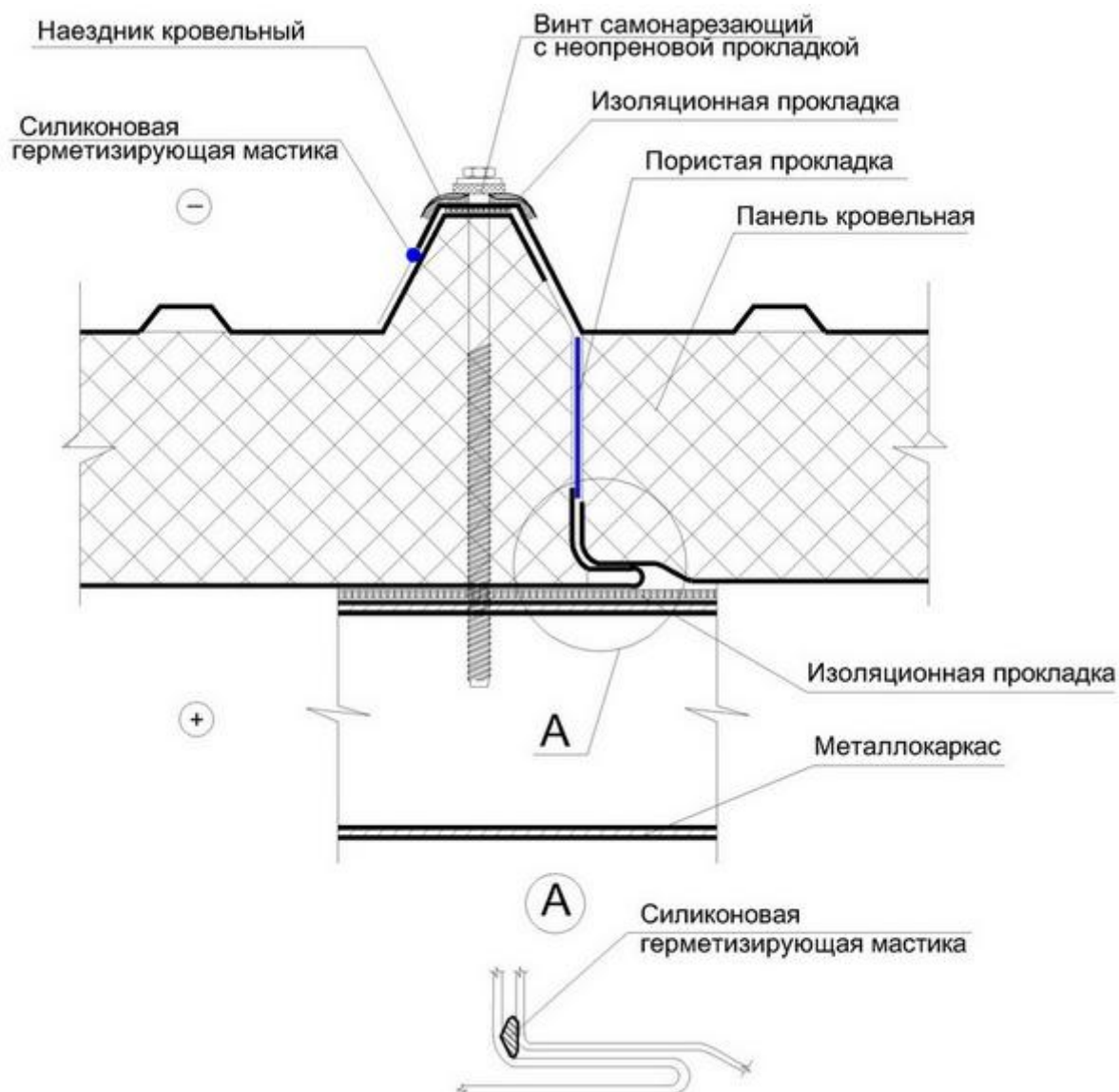
Рис. 1 Узел крепления панелей покрытия Изобуд с использованием кровельного наездника
